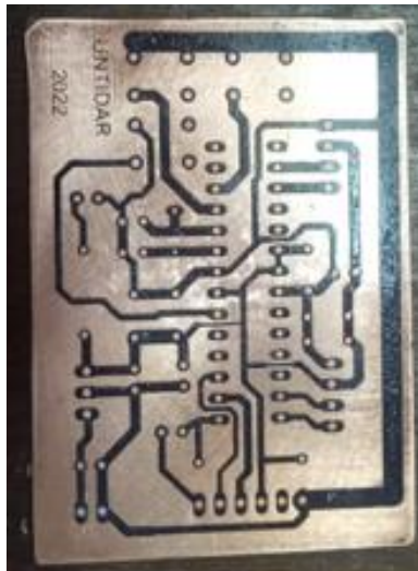
Gambar 5. Cetakan layout rangkaian pada PCB
