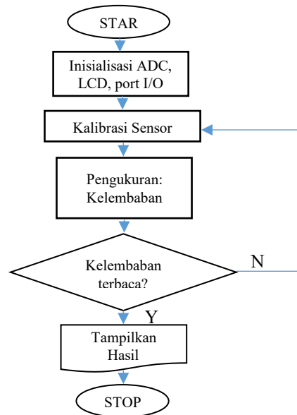
Gambar 3. Proses Pembuatan alat ukur kadar air biji kopi
